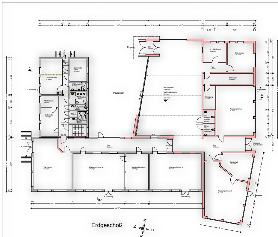
Grundriss: grau, bestehendes Gebäude, ausreichend für den Schulbeginn mit 2 Klassen; rot, Anbau für weitere 2 Klassen, Aula usw.
